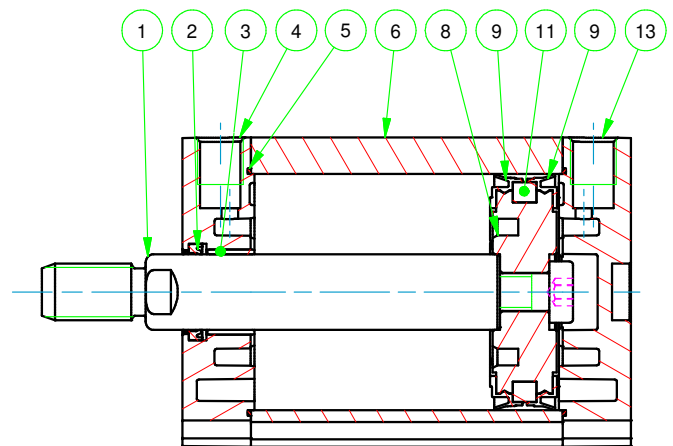
∅32 ÷ ∅125
