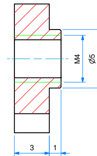
SEZ. "A-A"
